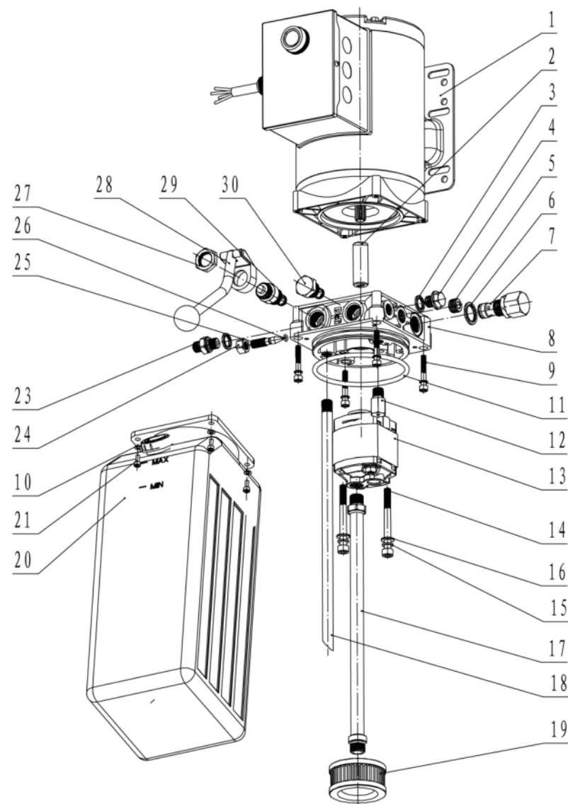
BN-2. 40PM-8-10b 泵站爆炸图
