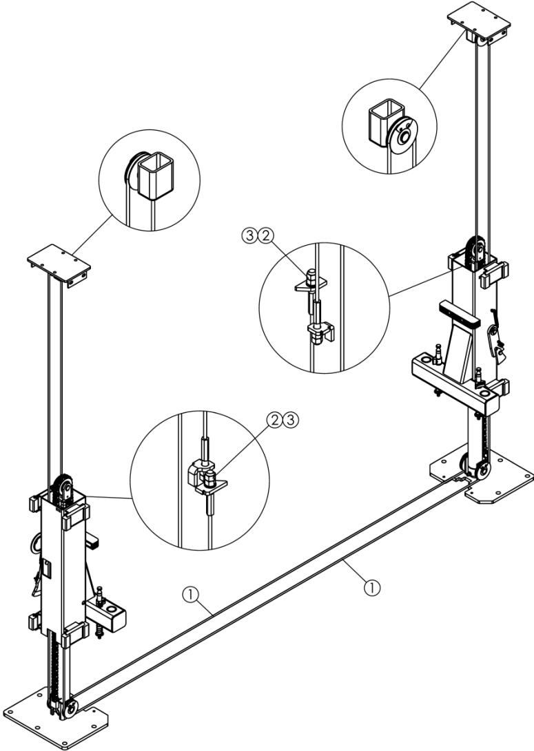
钢丝绳爆炸图
