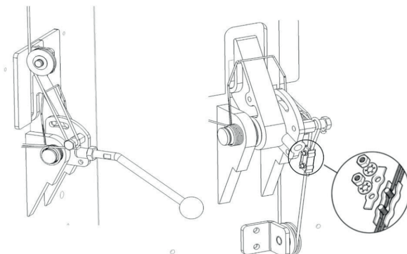
Стопорный механизм ведущей колонны
