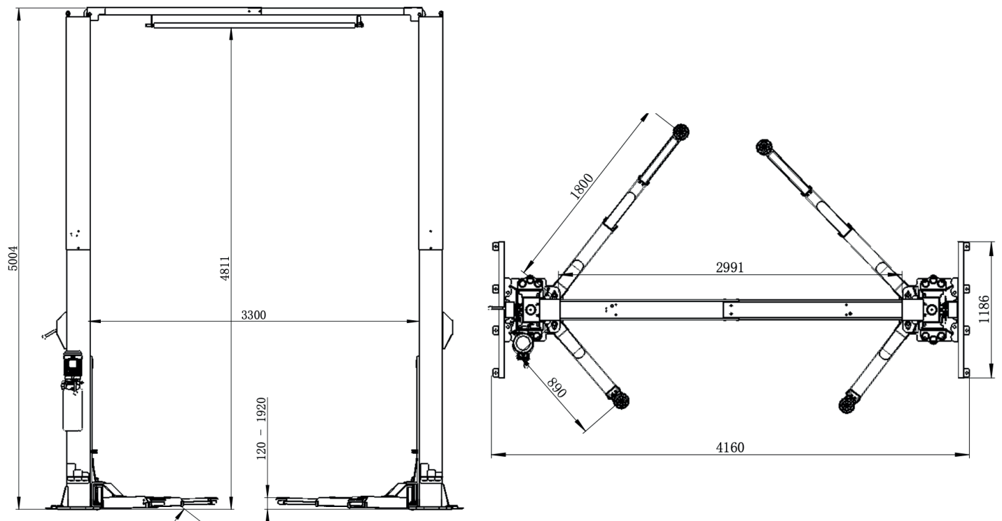
Установочный чертеж WDK-534
