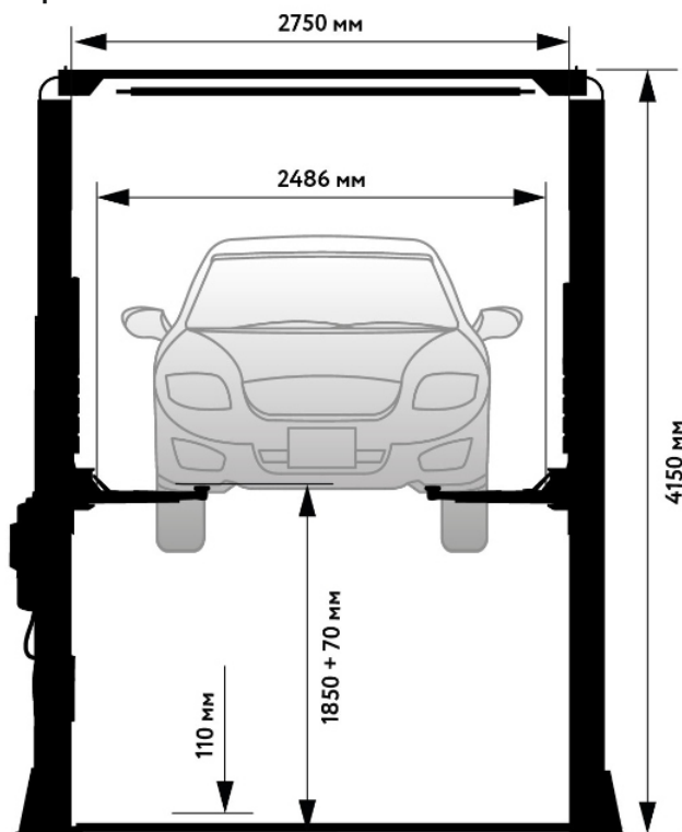
Чертеж WDK-529
