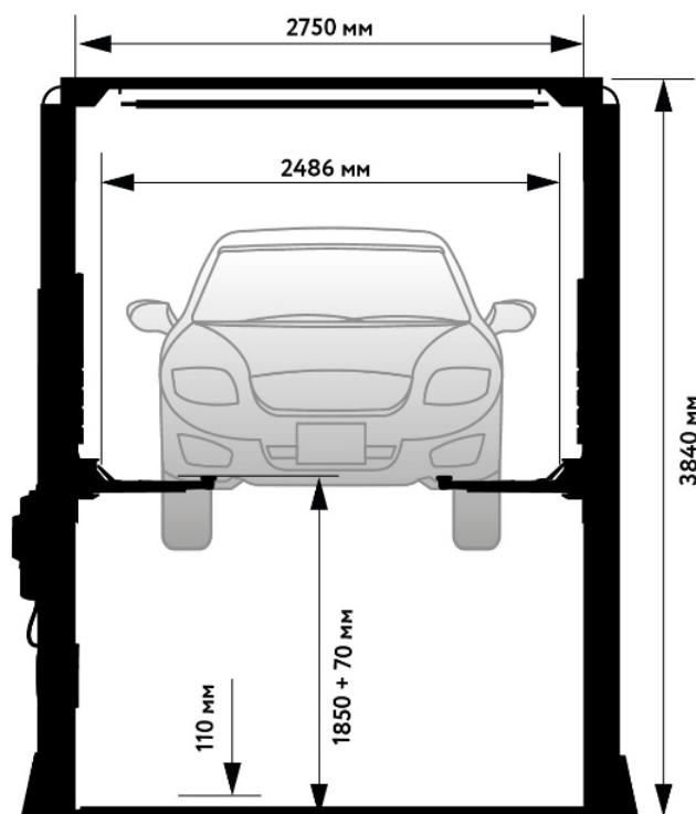
Чертеж WDK-529E
