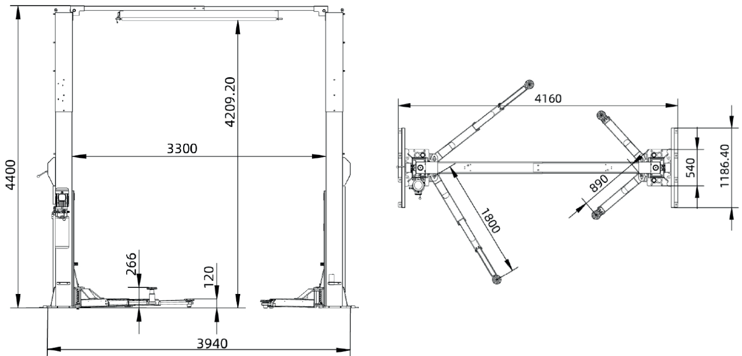
Чертеж подъемника WDK-525N
