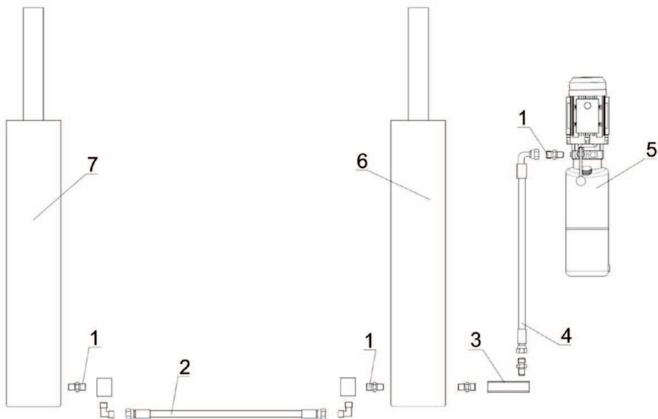
Гидравлическая схема WDK-524N
